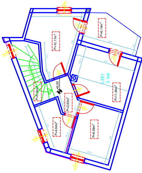
LAMELA 3 - 3.KAT. 43,62 m 2
