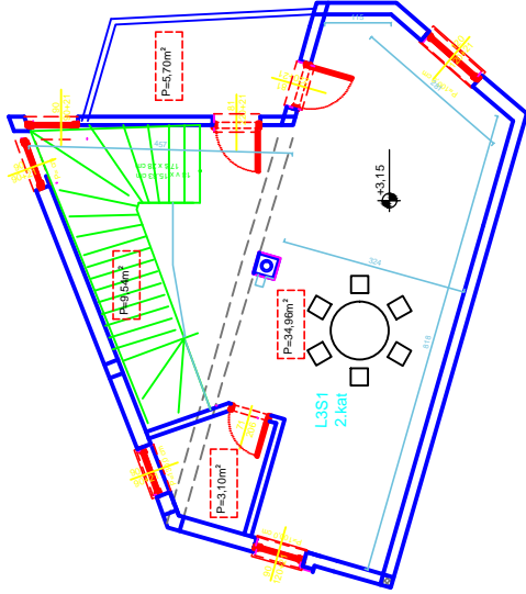
LAMELA 3 - 2.KAT. 47,60 m 2
